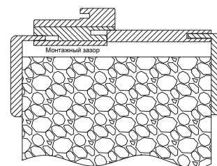
Схема сборки 3
